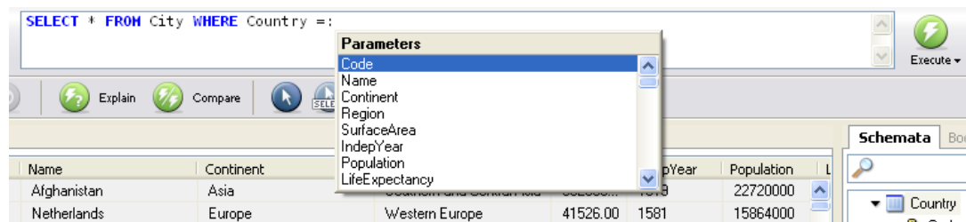
Figure 7.3. The dynamic parameter list
